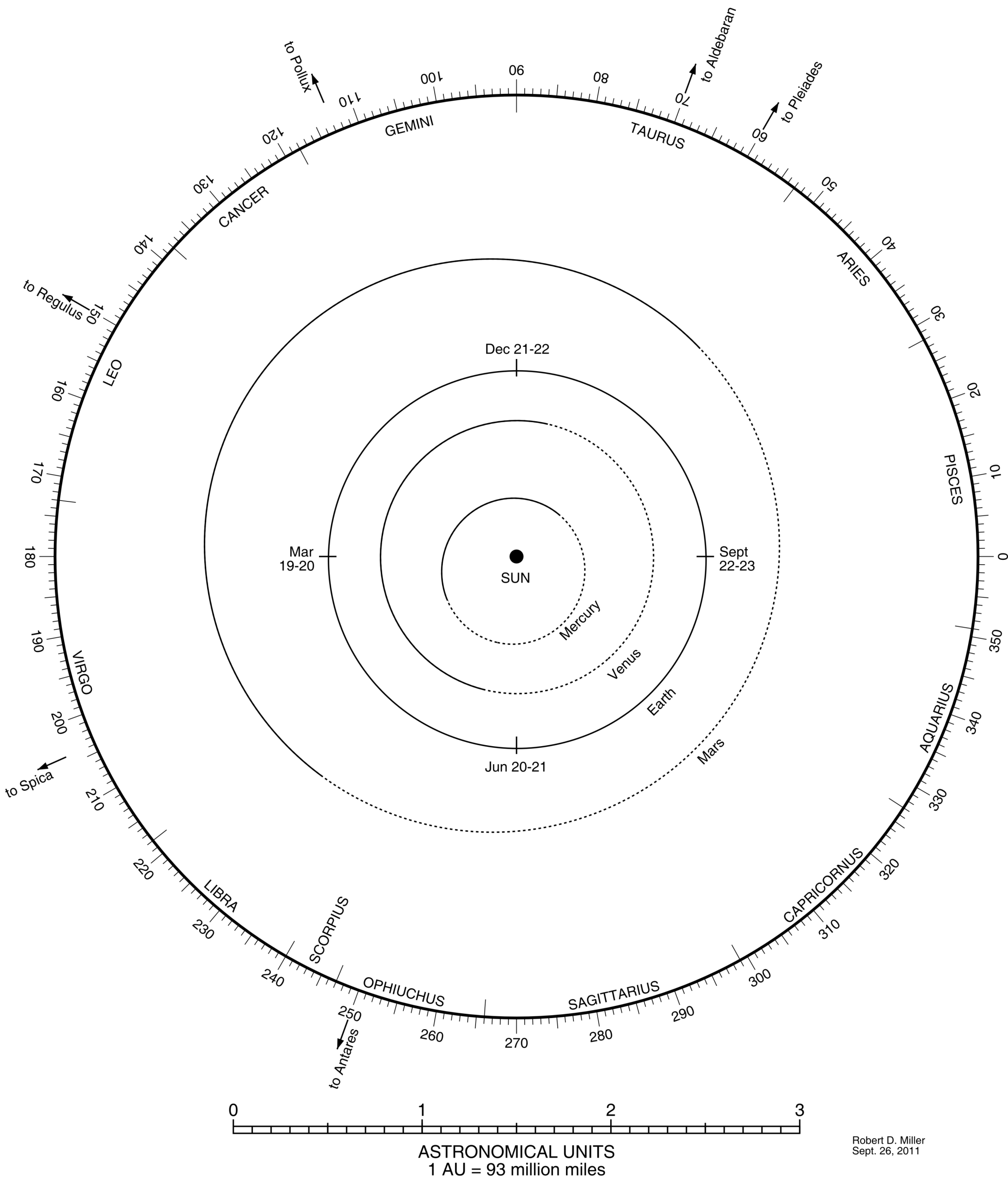
HELIOCENTRIC LONGITUDES OF THE PLANETS 2012—2013
